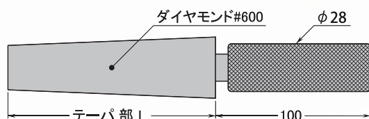
仕様寸法表 (単位:mm)
