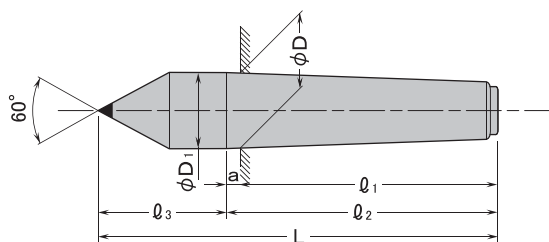
標準型仕様寸法表 (単位:mm)
