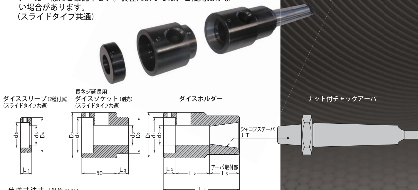
仕様寸法表 (単位:mm)
