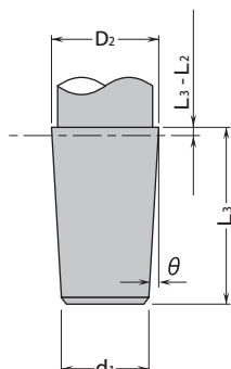
スピンドル側外径
